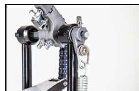
Sistema de mola com rolamento - regulagem de altura de sapata.
